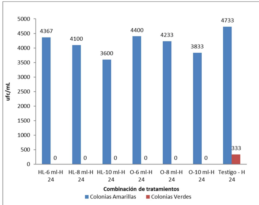
Figura 2. Promedios de número de colonias verdes y amarillas (ufc/mL) de Vibrio sp. a las 24 horas de aplicación de los extractos de Hierba luisa - HL ( Aloysia triphilla ) y Orégano - O ( Origanum vulgare ) a diferentes concentraciones (6, 8 y 10 mL/L).
